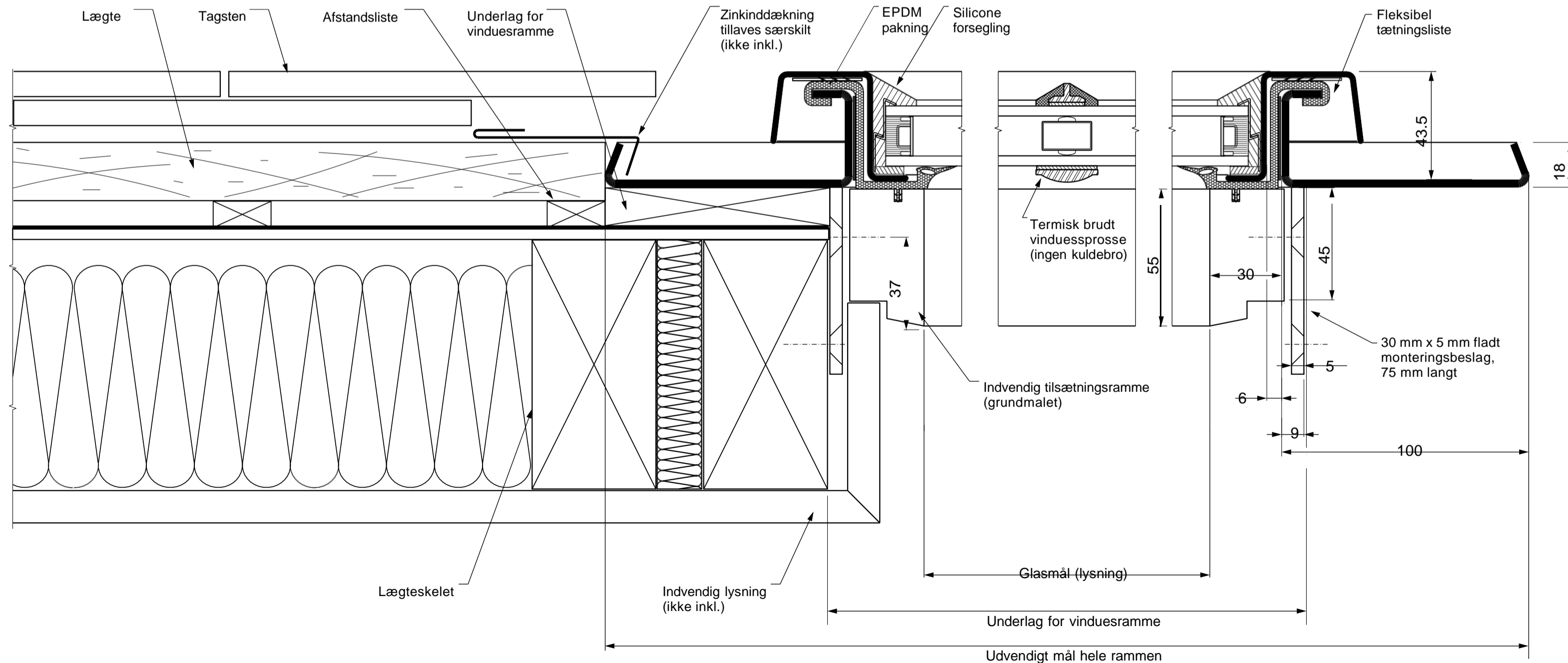
Snit A-A (1:1)
