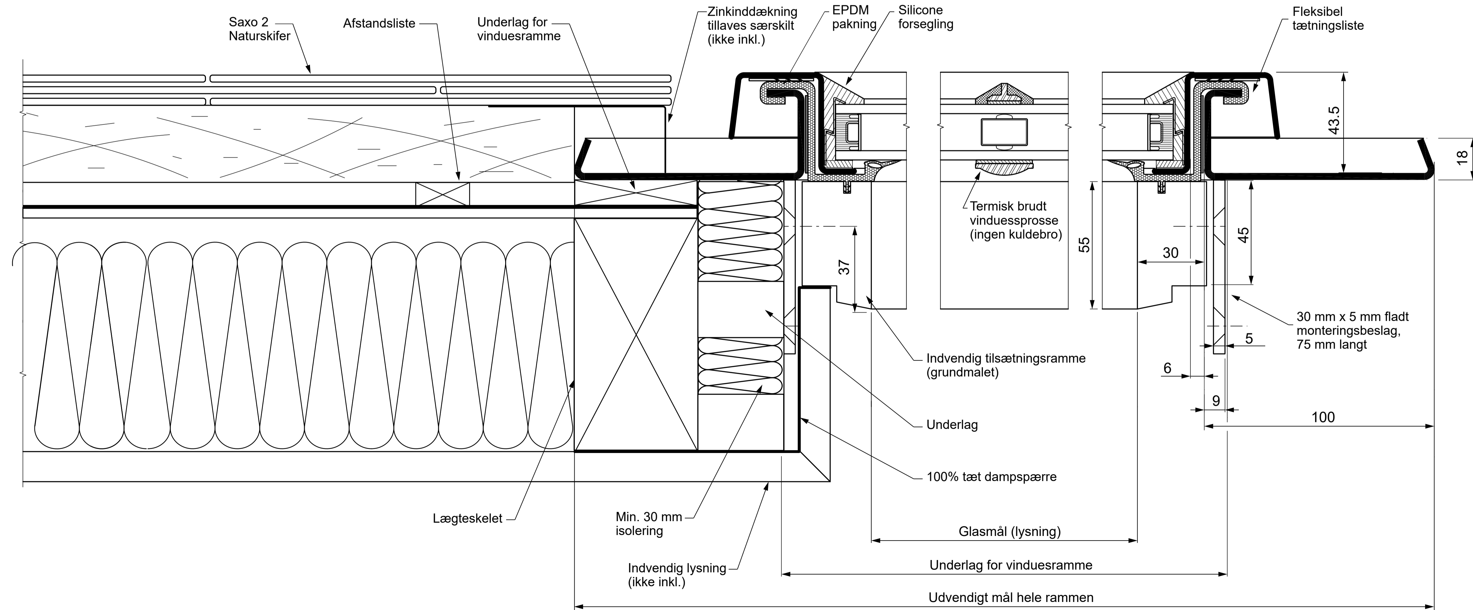
Snit A-A (1:1)
